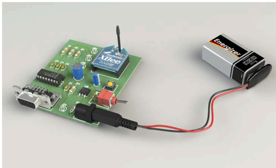
Figura 2.9: Placa de interface de comunicação.
