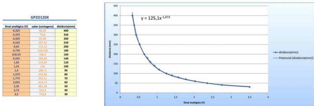
Figura 3.4: Gráfico dos valores do sinal analógico em função da distância do sensor GP2D120.
